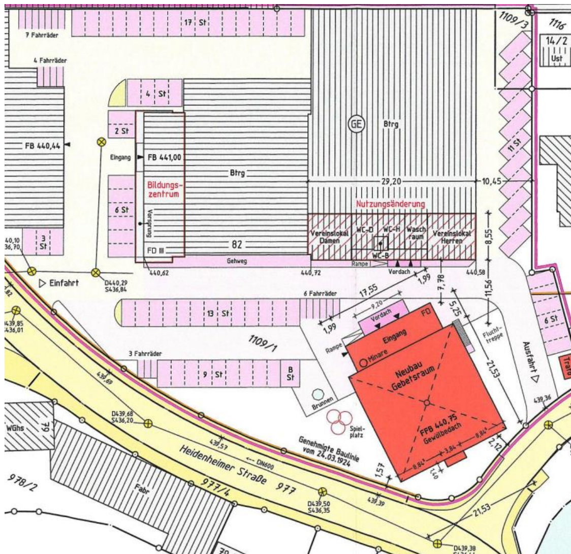
(Lageplan)
